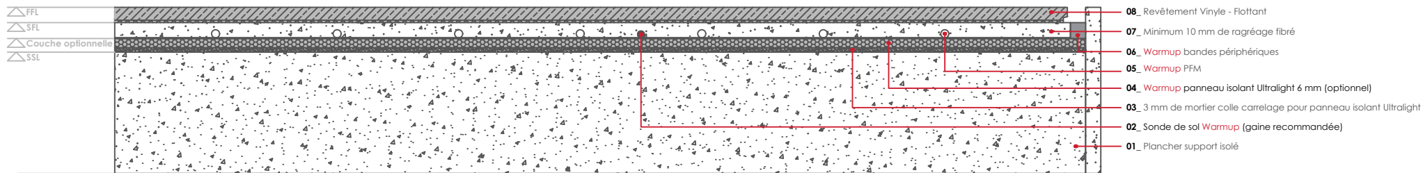
WARMUP PFM SYSTÈME. Revêtement Vinyle - Flottant
