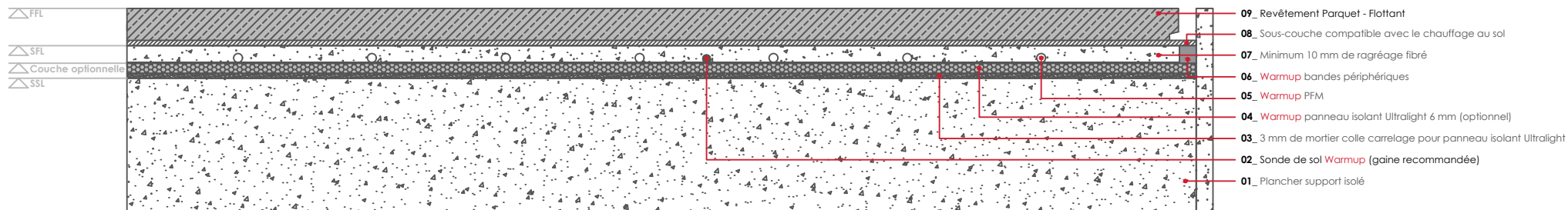
WARMUP PFM SYSTÈME. Revêtement Parquet - Flottant
