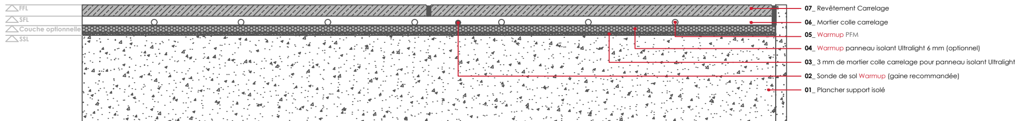
WARMUP PFM SYSTÈME. Revêtement Carrelage
