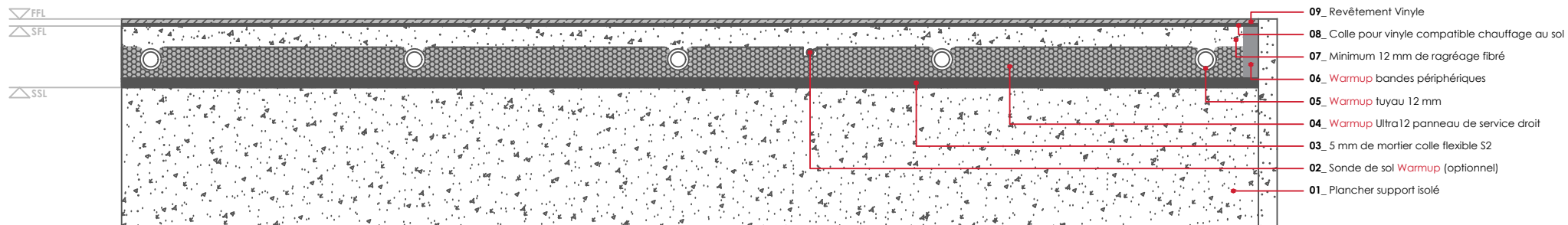
WARMUP ULTRA12 SYSTÈME. Revêtement Vinyle - Collé
