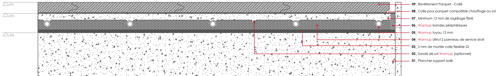
WARMUP ULTRA12 SYSTÈME. Revêtement Parquet - Collé
