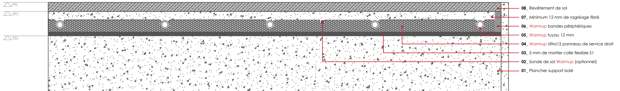
WARMUP ULTRA12 SYSTÈME. Installation Standard
