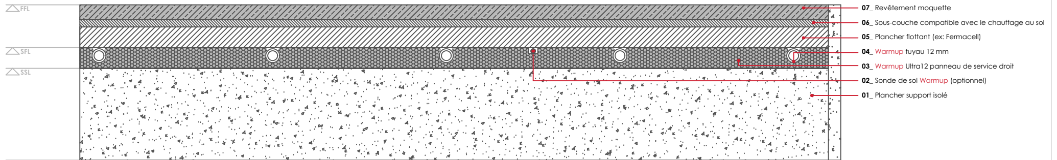
WARMUP ULTRA12 SYSTÈME. Revêtement Moquette
