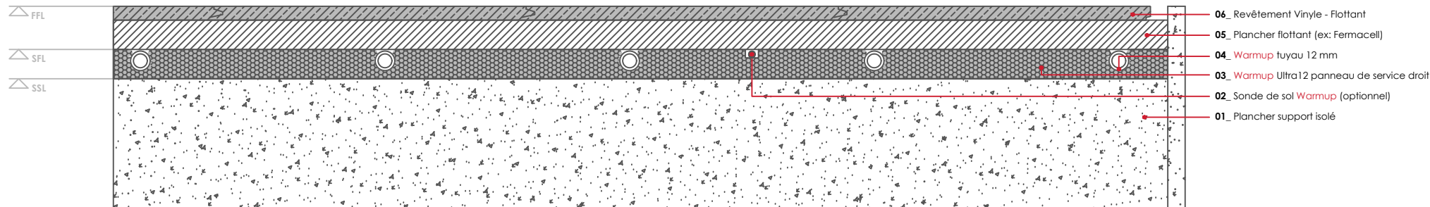
WARMUP ULTRA12 SYSTÈME. Revêtement Vinyle - Flottant
