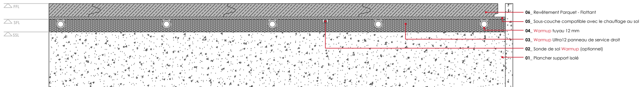
WARMUP ULTRA12 SYSTÈME. Revêtement Parquet - Flottant
