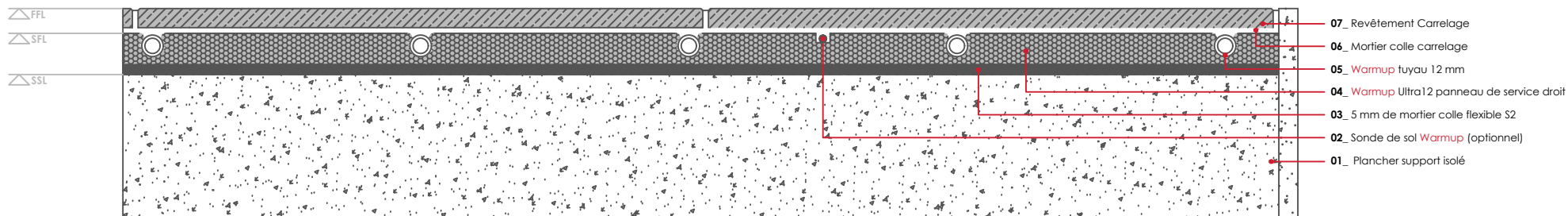
WARMUP ULTRA12 SYSTÈME. Revêtement Carrelage
