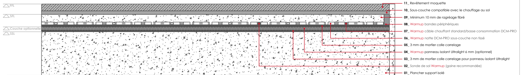
WARMUP DCM-PRO SYSTÈME. Revêtement Moquette
