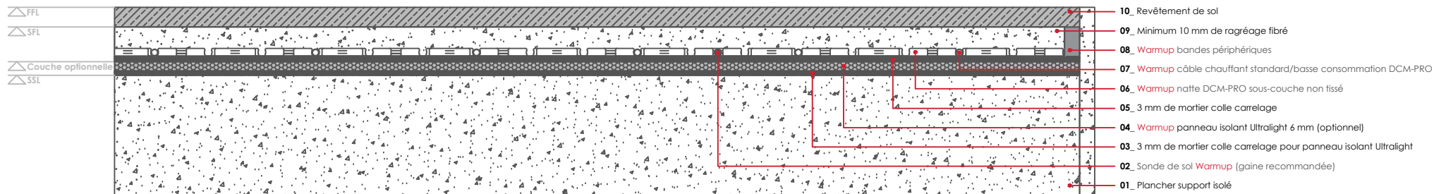
WARMUP DCM-PRO SYSTÈME. Installation Standard
