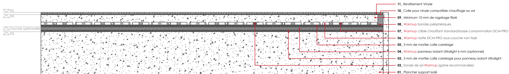
WARMUP DCM-PRO SYSTÈME. Revêtement Vinyle - Collé
