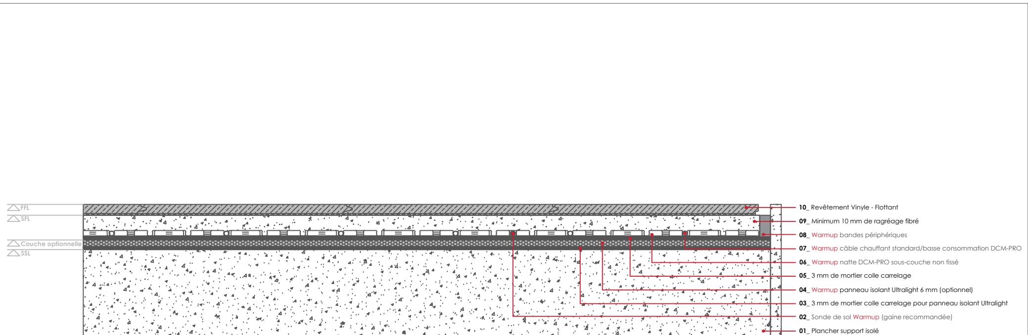
WARMUP DCM-PRO SYSTÈME. Revêtement Vinyle - Flottant
