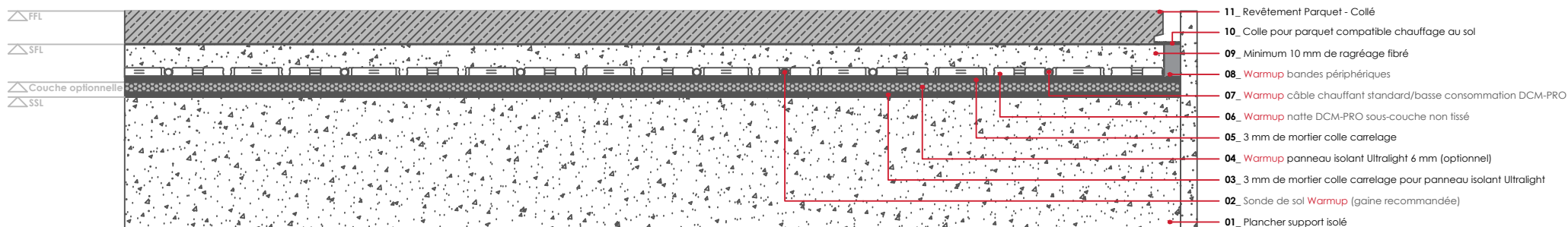
WARMUP DCM-PRO SYSTÈME. Revêtement Parquet - Collé
