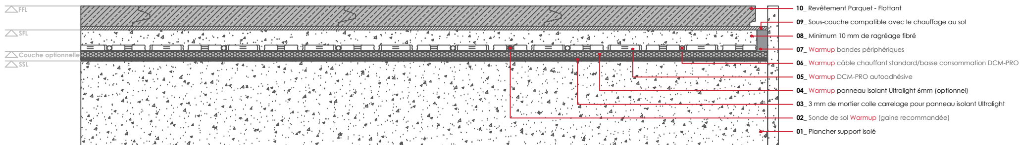
WARMUP DCM-PRO SYSTÈME. Revêtement Parquet - Flottant
