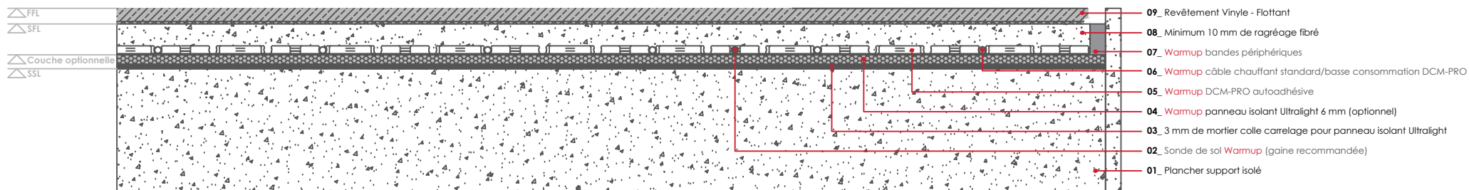
WARMUP DCM-PRO SYSTÈME. Revêtement Vinyle - Flottant
