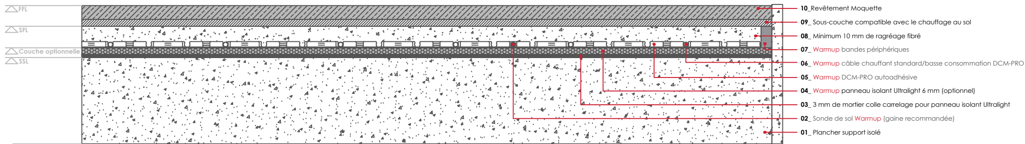
WARMUP DCM-PRO SYSTÈME. Revêtement Moquette
