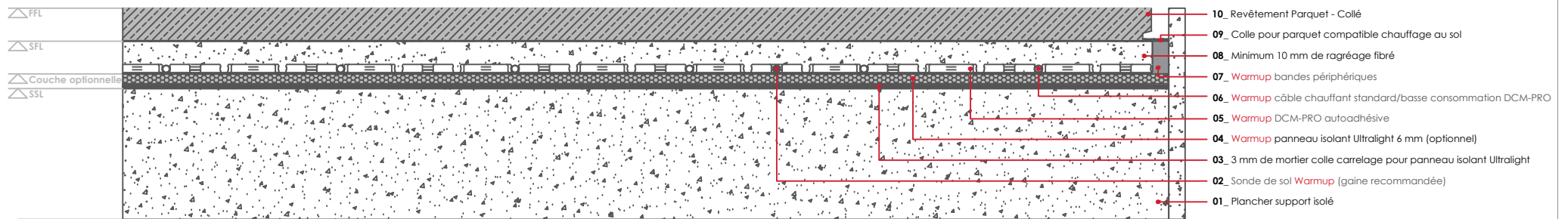
WARMUP DCM-PRO SYSTÈME. Revêtement Parquet - Collé
