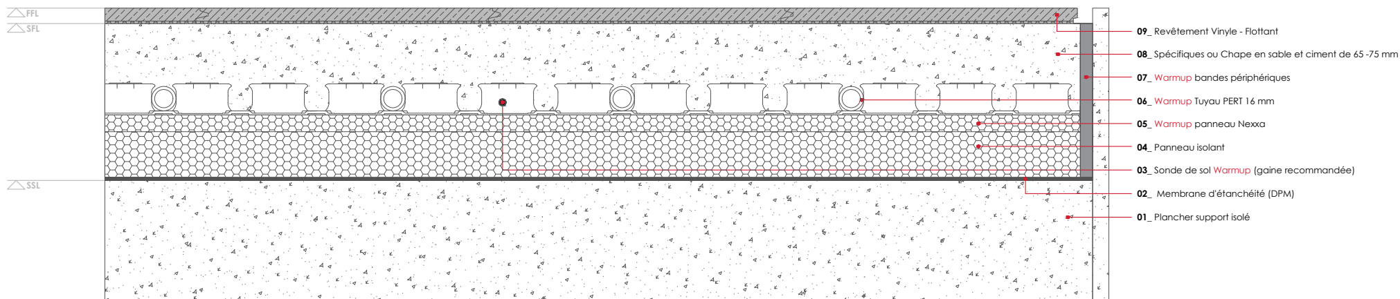
WARMUP NEXXA SYSTÈME. Revêtement Vinyle - Flottant
