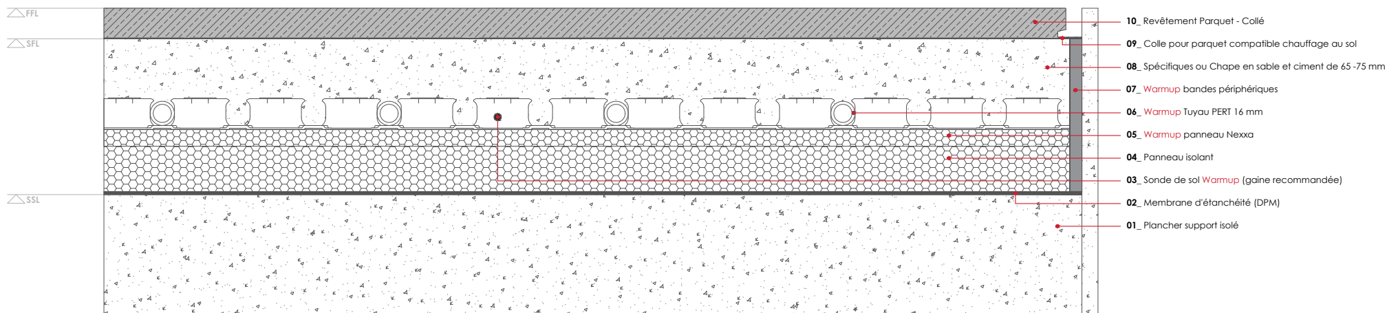
WARMUP NEXXA SYSTÈME. Revêtement Parquet - Collé
