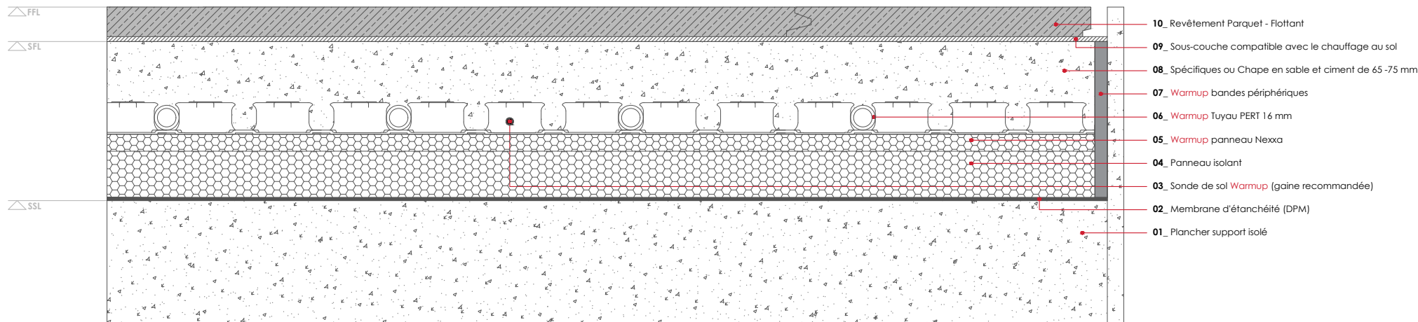
WARMUP NEXXA SYSTÈME. Revêtement Parquet - Flottant
