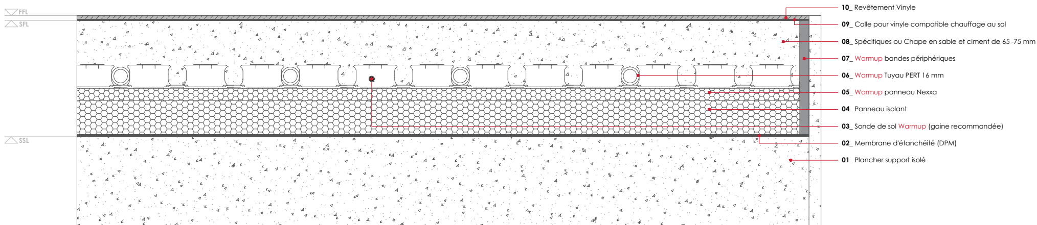
WARMUP NEXXA SYSTÈME. Revêtement Vinyle - Collé
