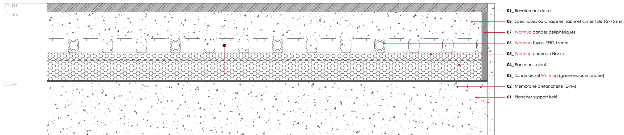
WARMUP NEXXA SYSTÈME. Installation Standard
