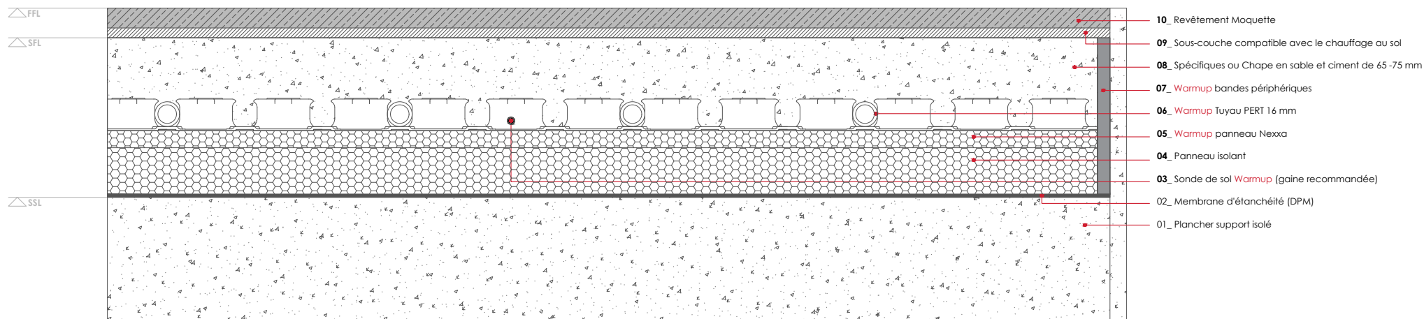
WARMUP NEXXA SYSTÈME. Revêtement Moquette
