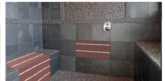
Trame chauffante 12V en espace hammam
